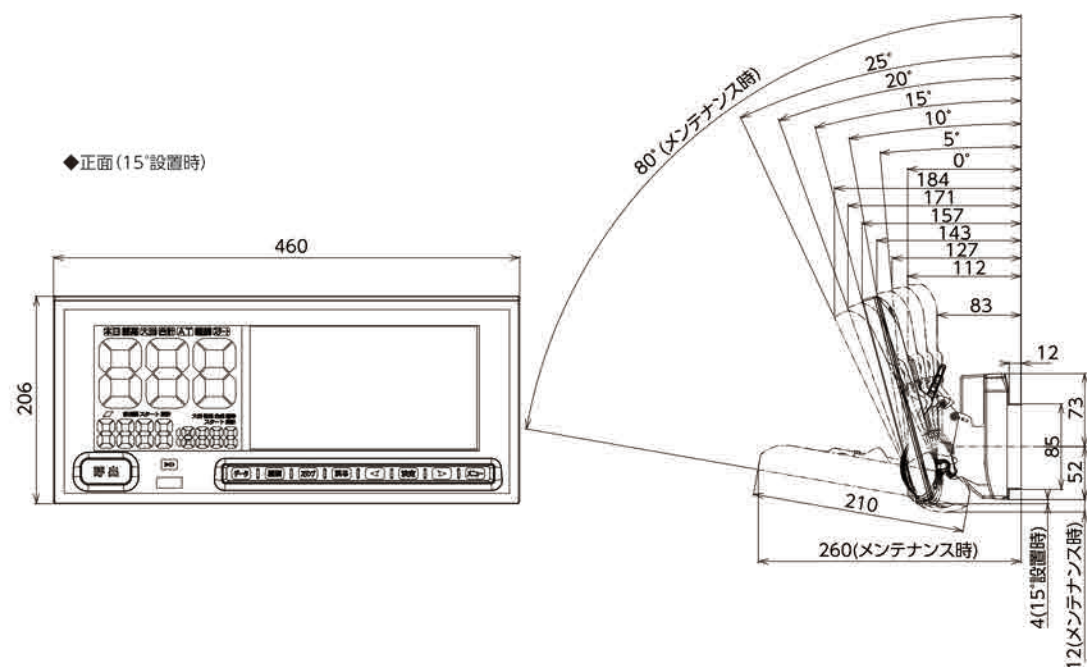
取付ベース寸法図 (mm)
