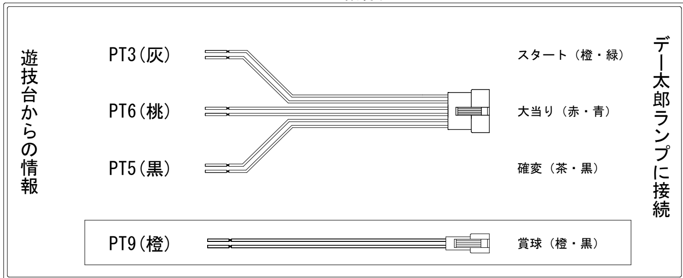
外部端子板
