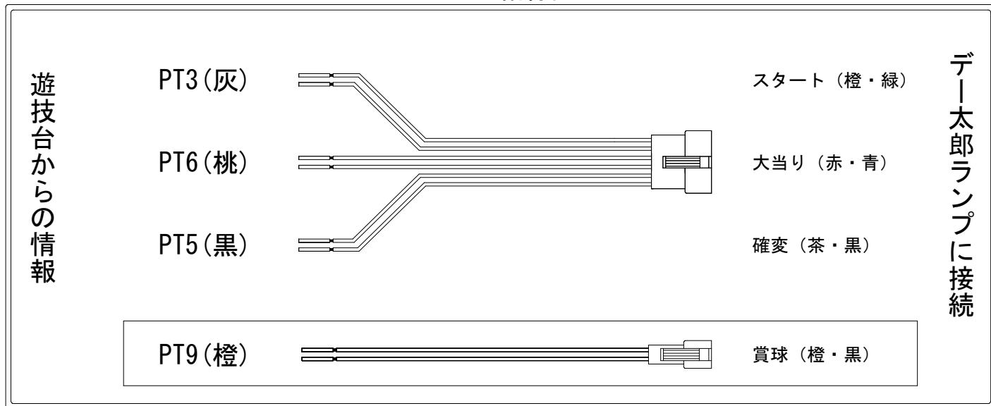
外部端子板
