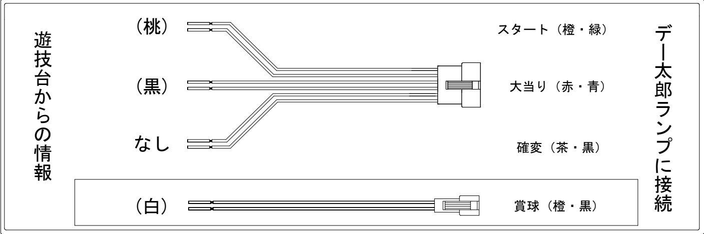
ハーネス結線図
