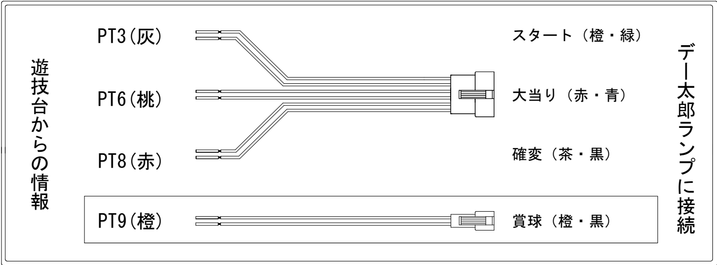
外部端子板
