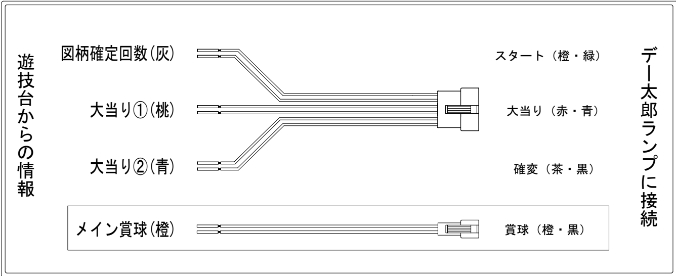
外部端子板
