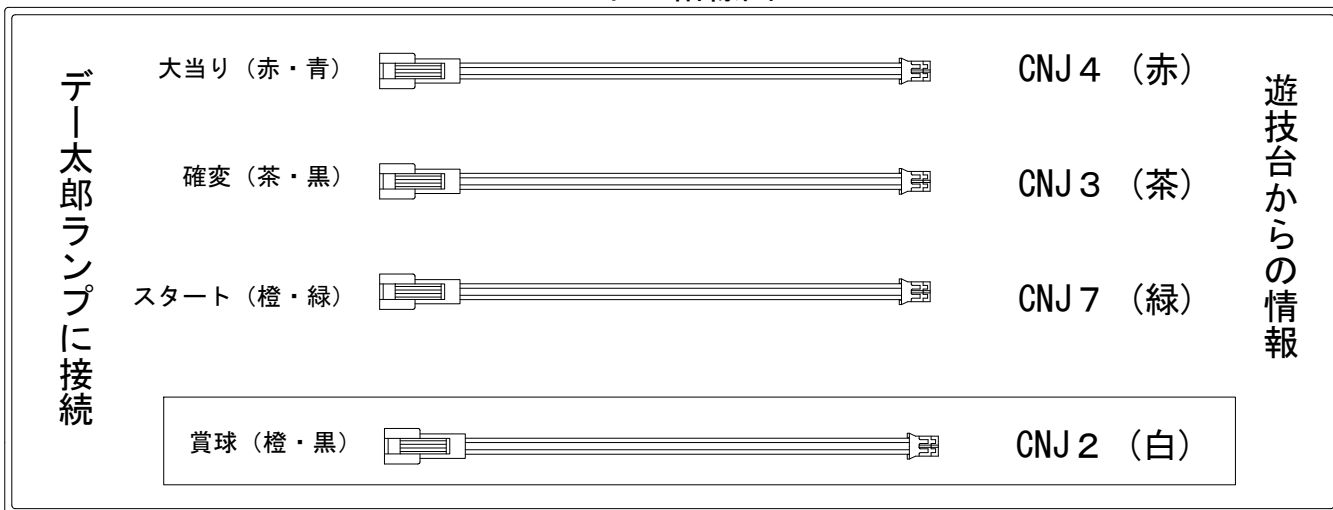
外部端子板
