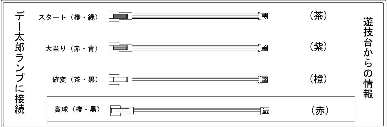
外部端子板
