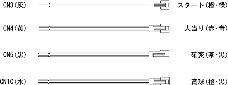
ハーネス結線図
