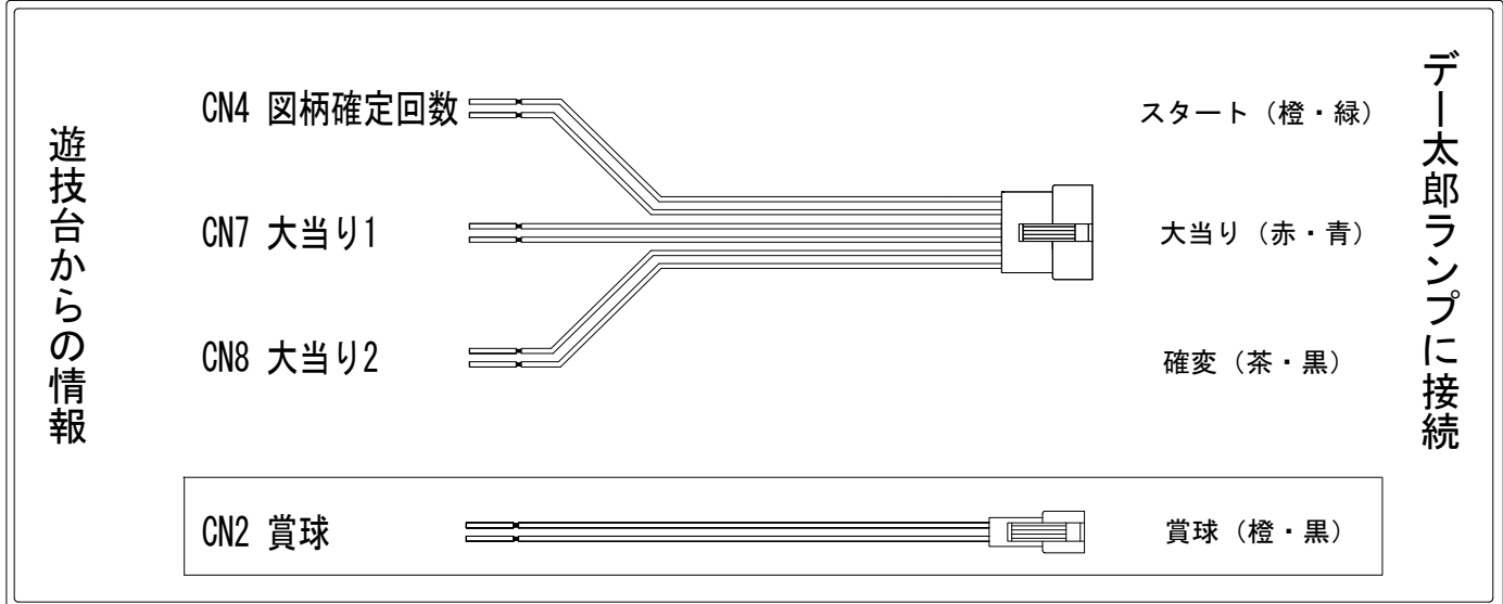
外部端子板
