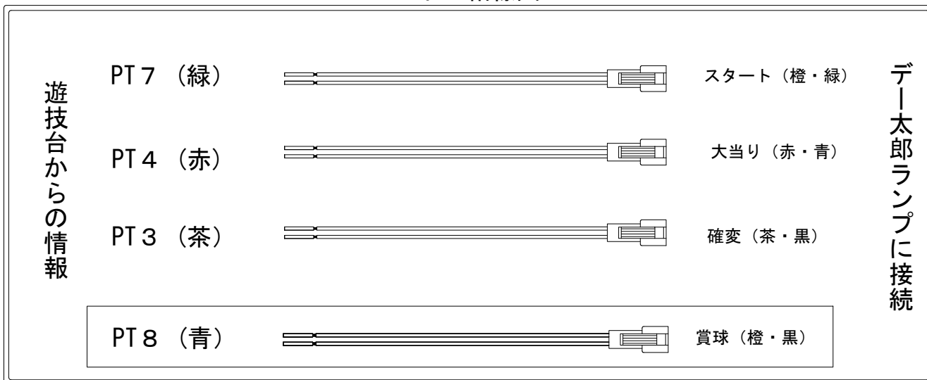
外部端子板
